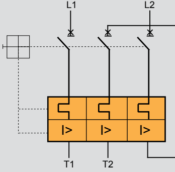
Bağlantı şeması
