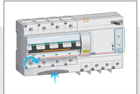
BAĞLANTILARI SIKMAK ve bağlantı noktasına koruyucuyu bağlamak
